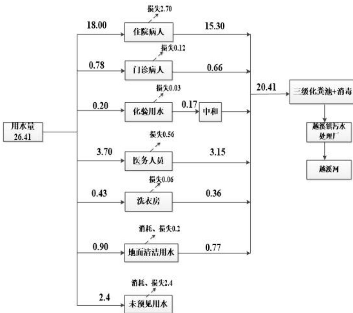
图 2-1 水平衡示意图 m³/d
