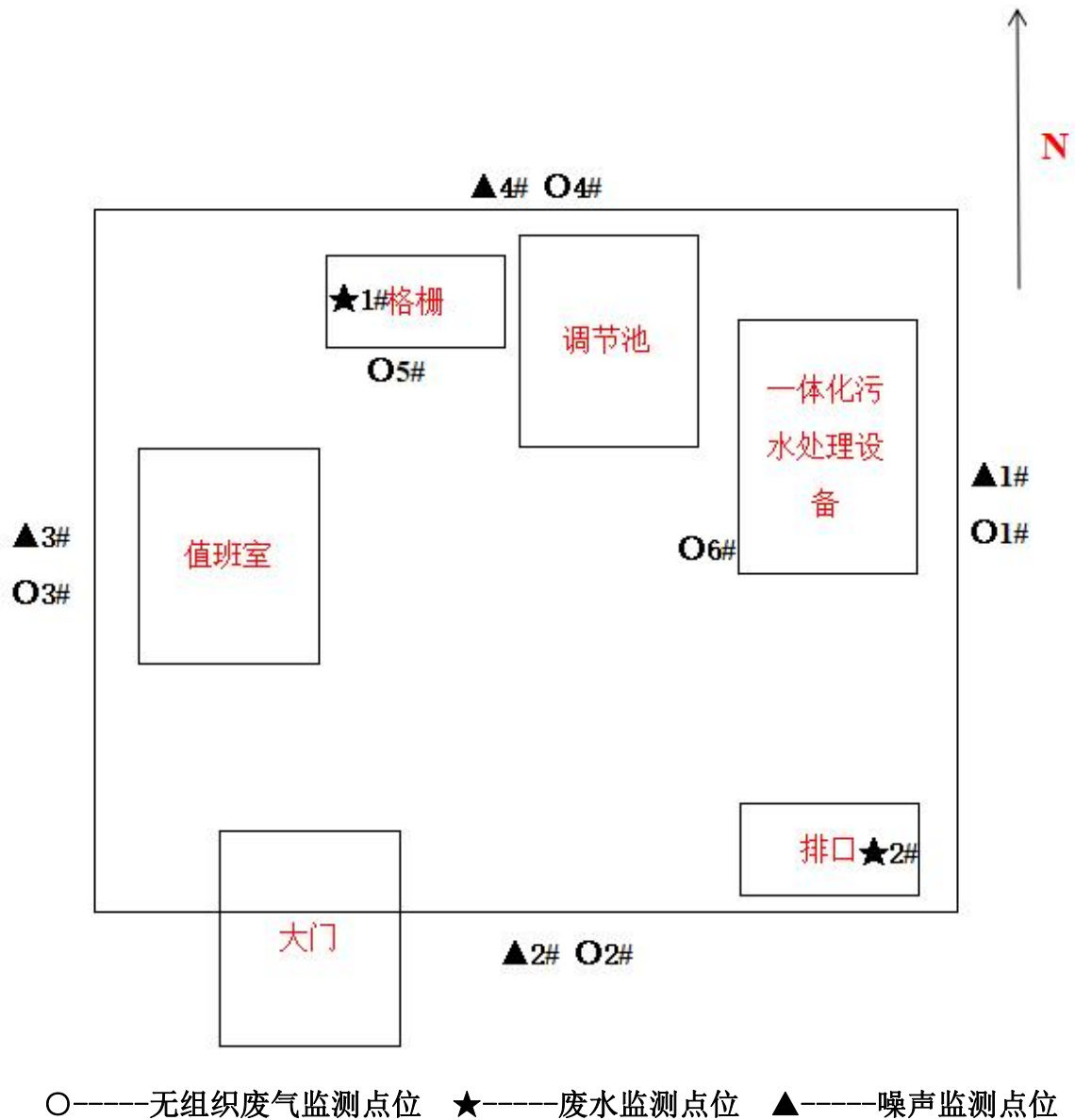
附图2 平面布置及监测点位图
