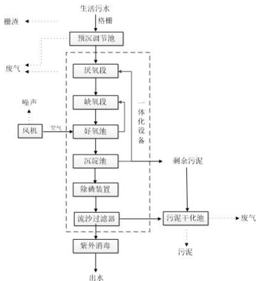
图 2-1 工艺流程及产污环节图
